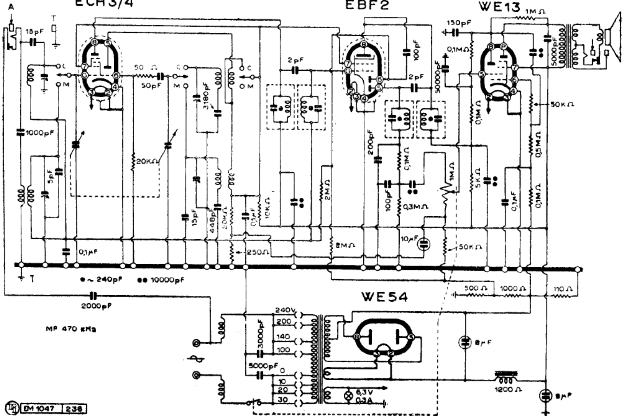
Lo schema elettrico del mod. "Phonola 407..."
